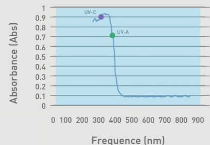
Absorption spectra of TiO 2
