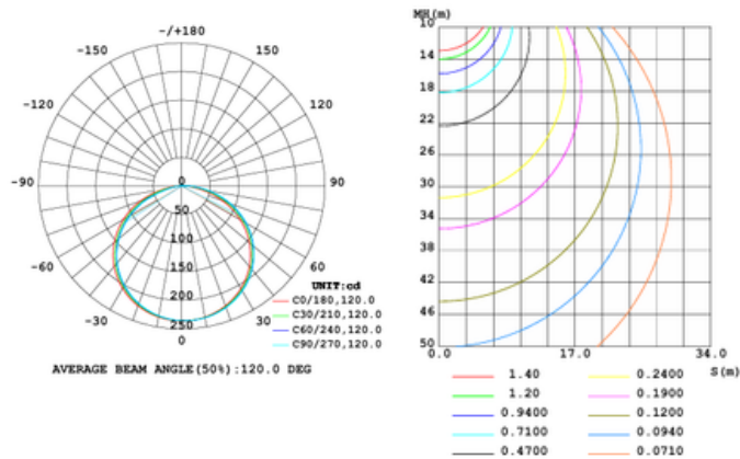
Valonjakokäyrä
